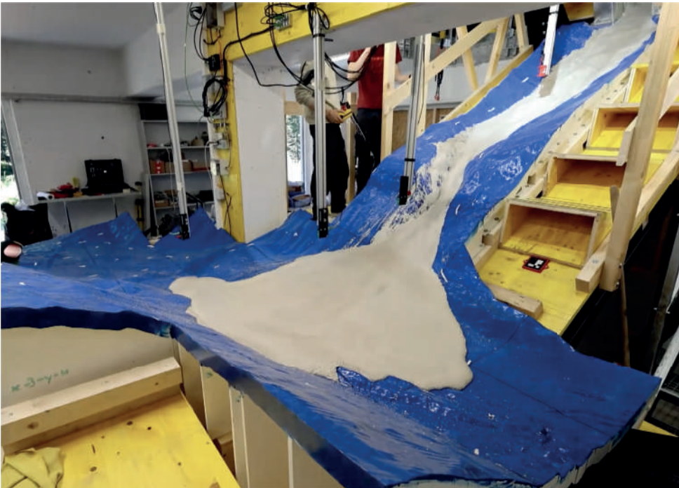
Le modèle tridimensionnel de l'effondrement de Blatten. Extrait du 19:20 de la RTS.
